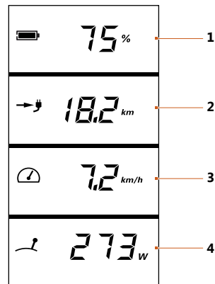
Fig. 59: Panoramica del display multifunzione
