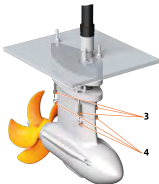
Fig. 34: Démontage du moteur
