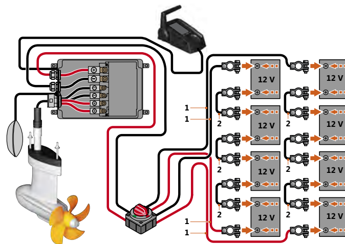
Fig. 18: Schéma électrique des batteries au plomb
