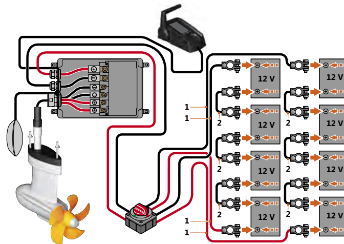
Fig. 57: Schema elettrico batterie al piombo
