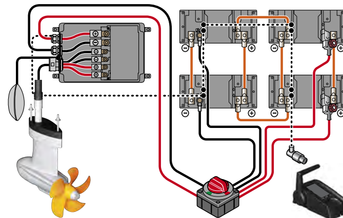
Fig. 16: Schéma électrique de la Power 26-104
