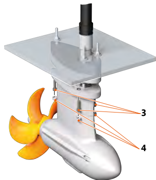
Fig. 73: Smontaggio del motore
