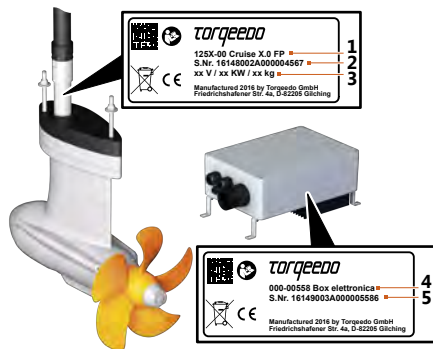
Fig. 40: Targhette del motore e del box elettronica
