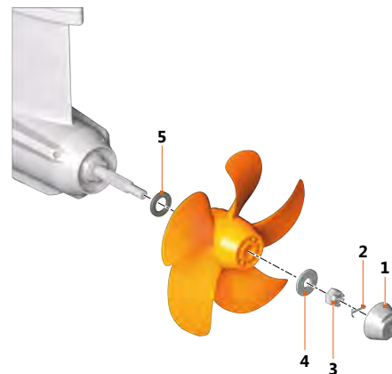
Fig. 36: Fixation de l'hélice
