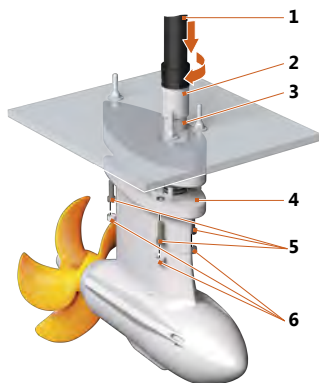
Fig. 35: Montage du moteur
