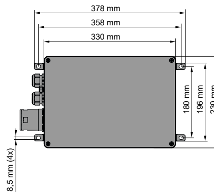
Fig. 13: Dimensions du boîtier électronique
