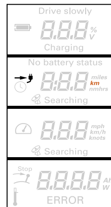
Fig. 63: Display multifunzione, menu Setup
