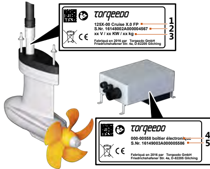
Fig. 1: Plaques signalétiques du moteur et du boîtier électronique
