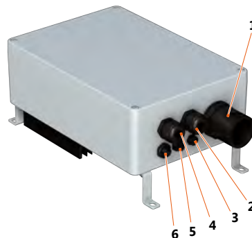
Fig. 15: Branchements du boîtier électronique
