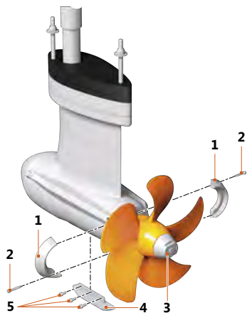
Fig. 38: Anodes
