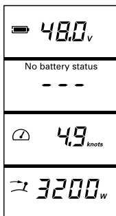
Fig. 61: Display multifunzione senza setup
