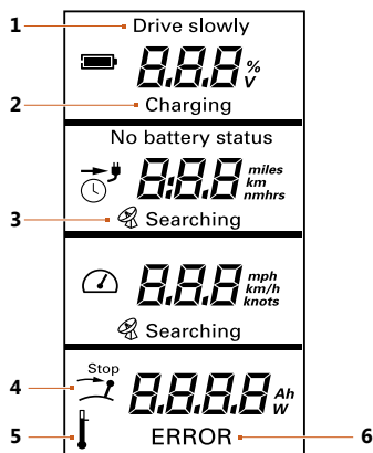
Fig. 60: Display multifunzione, menu Setup
