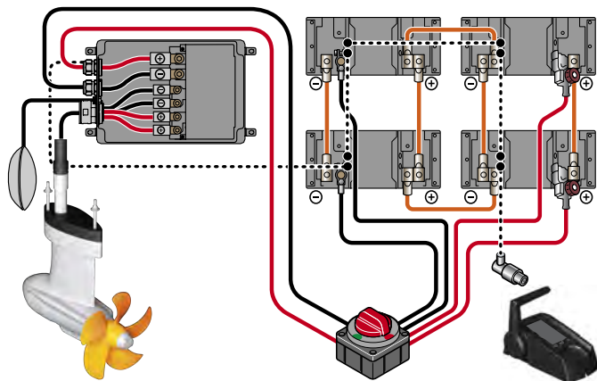
Fig. 55: Schema elettrico Power 26-104
