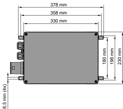
Fig. 52: Misure del box elettronica
