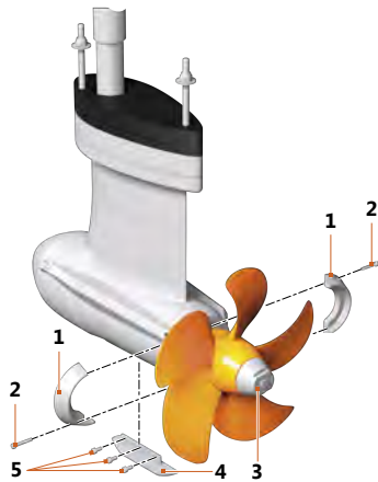
Fig. 77: Anodi
