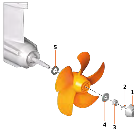
Fig. 75: Fissaggio dell'elica
