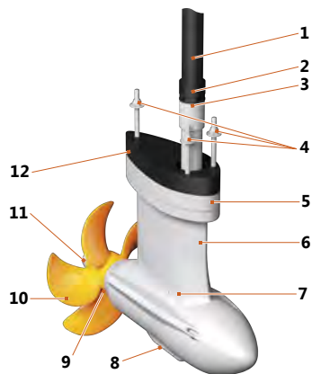
Fig. 8: Liste des pièces du système de propulsion et des composants
