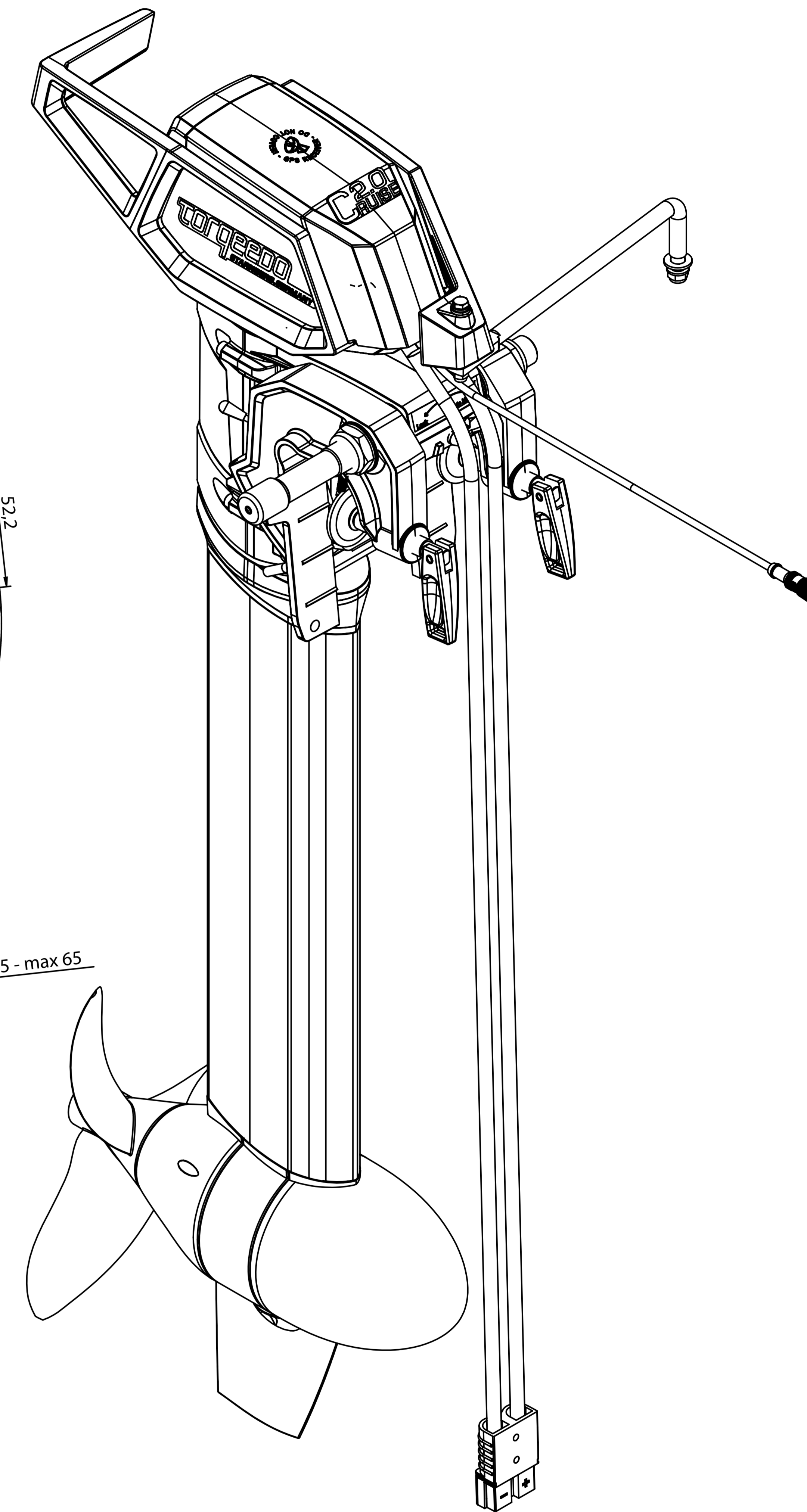
DETAIL Z MAßSTAB 1 : 1
