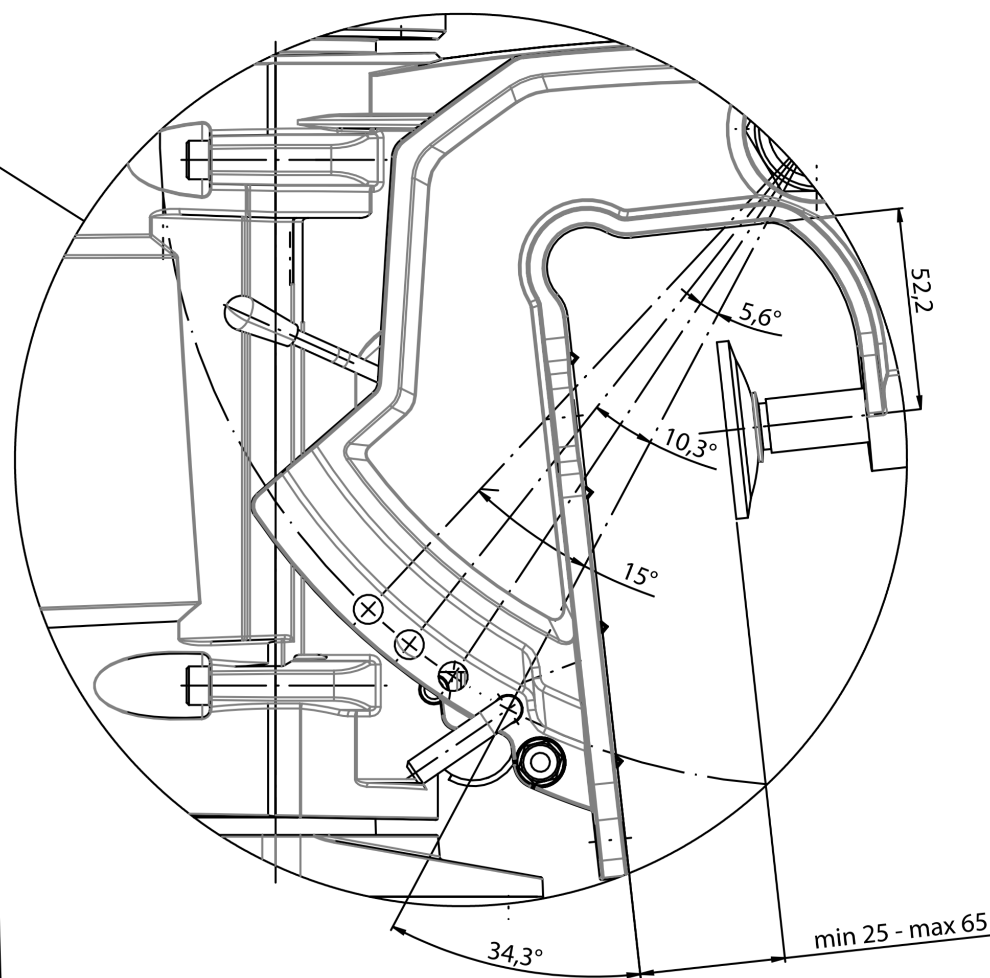
DETAIL Z MAßSTAB 1 : 1
