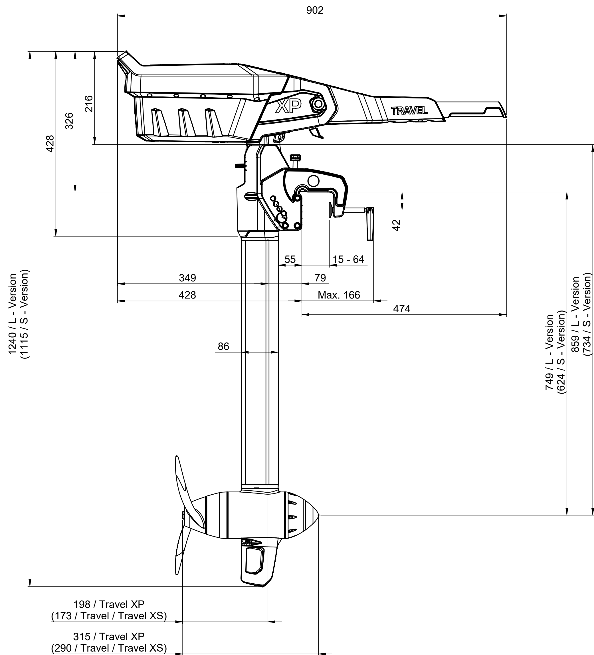
Side View / Seitenansicht
