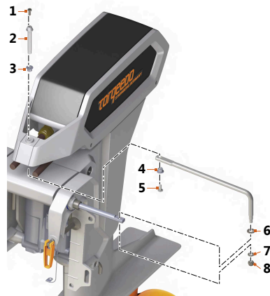
Fig. 36: Éléments de la commande à distance
