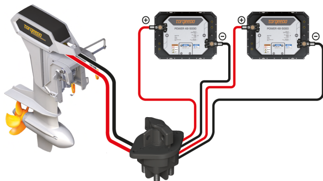
Fig. 14: Schema elettrico Power 48-5000
