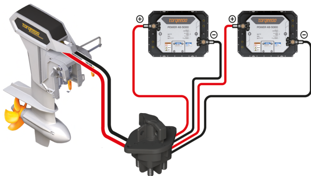
Fig. 42: Schéma électrique de la Power 48-5000
