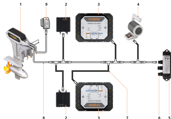
Fig. 39: Structure schématique d'un réseau TorqLink avec la manette de commande 1949-1952
