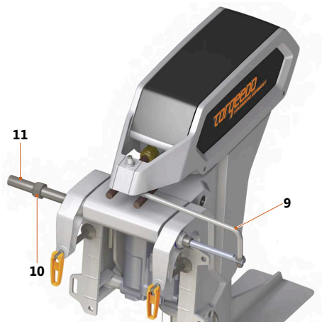
Fig. 37: Commande à distance
