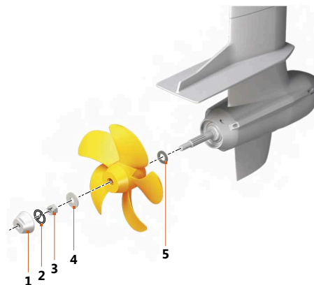
Fig. 35: Fixation de l'hélice
