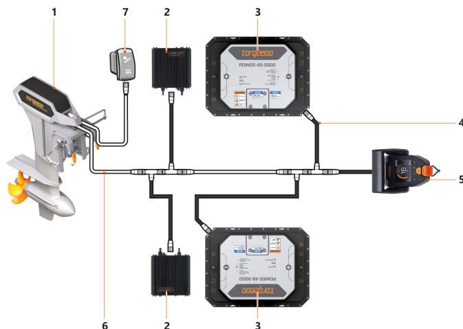
Fig. 38: Structure schématique d'un réseau TorqLink avec la manette de commande 1976-00
