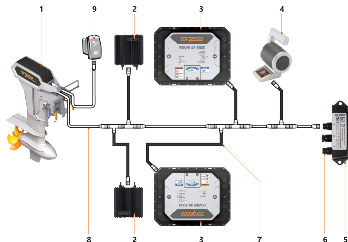
Fig. 11: Struttura schematica di una rete TorqLink con la leva dell'acceleratore 1949-1952
