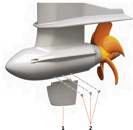
Fig. 34: Fixation de la dérive
