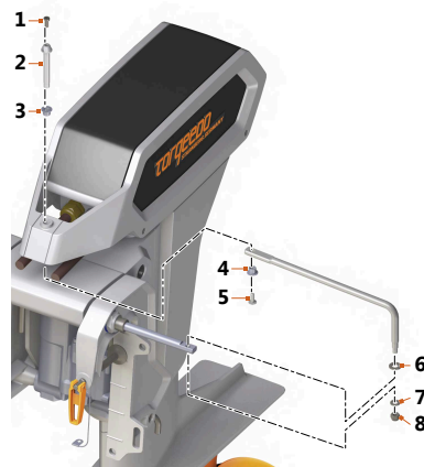
Fig. 8: Componenti del comando dello sterzo a distanza
