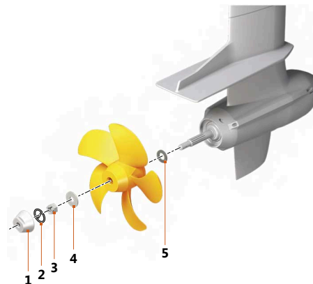
Fig. 7: Fissaggio dell'elica
