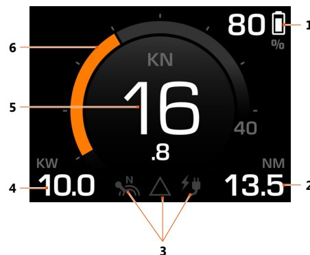
Fig. 49: Vista geral do visor multifunções
