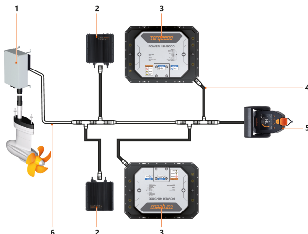
Fig. 45: Estrutura esquemática de uma rede TorqLink com a alavanca do acelerador remoto 1976-00
