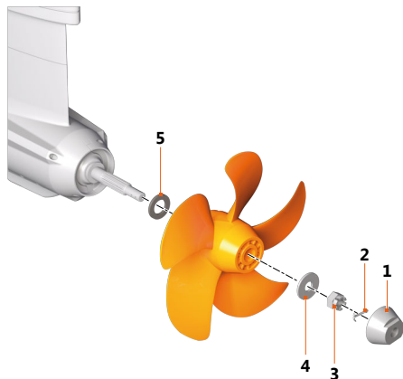
Fig. 27: Fijación de la hélice
