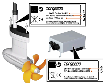
Fig. 31: Placas de identificação do motor e da caixa eletrônica
