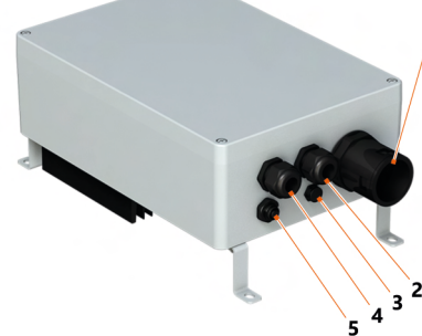
Fig. 14: Conexiones del cuadro electrónico
