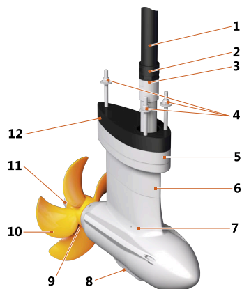
Fig. 36: Vista geral de elementos de transmissão e componentes
