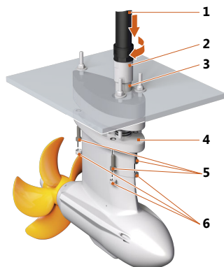
Fig. 39: Montagem do motor
