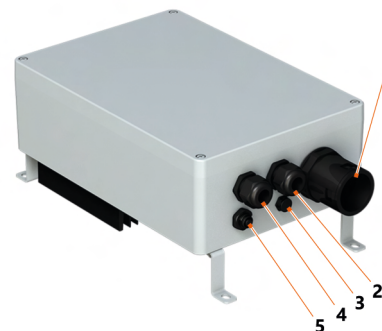
Fig. 44: Ligações da caixa eletrônica
