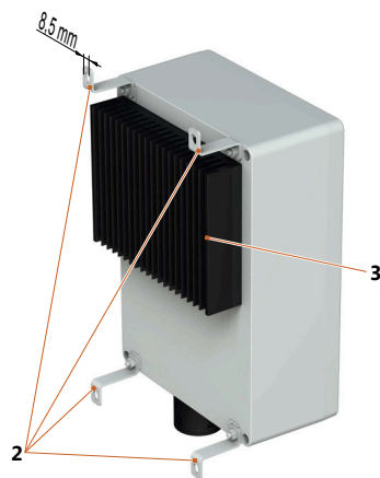
Fig. 43: Posição de fixação da caixa eletrônica
