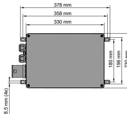
Fig. 42: Dimensões da caixa eletrónica
