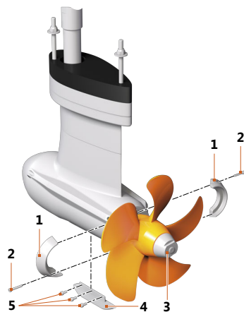
Fig. 29: Ánodos
