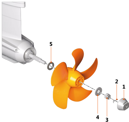
Fig. 57: Fixação da hélice
