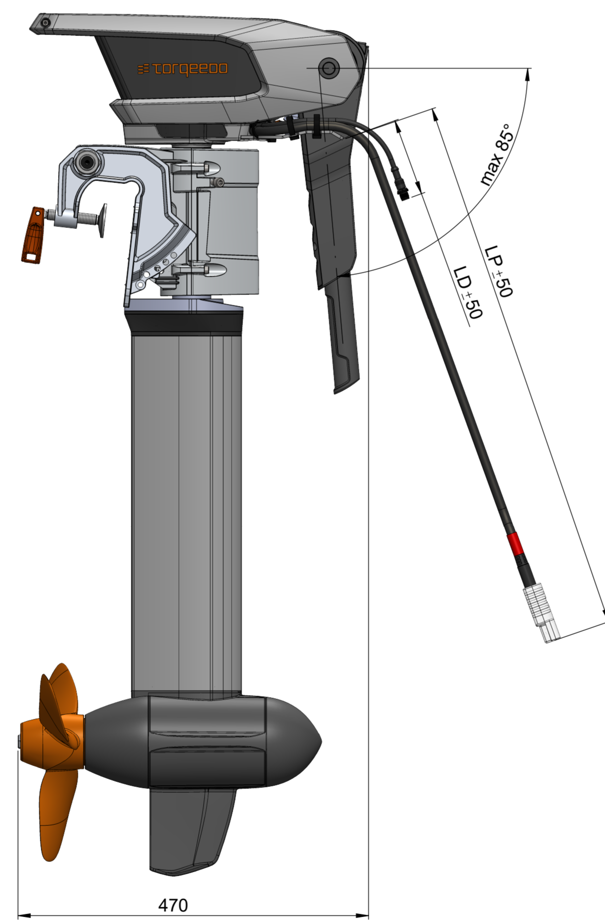
Transport Position Spiegelhalterung 180° gedreht transom mount turned 180°
