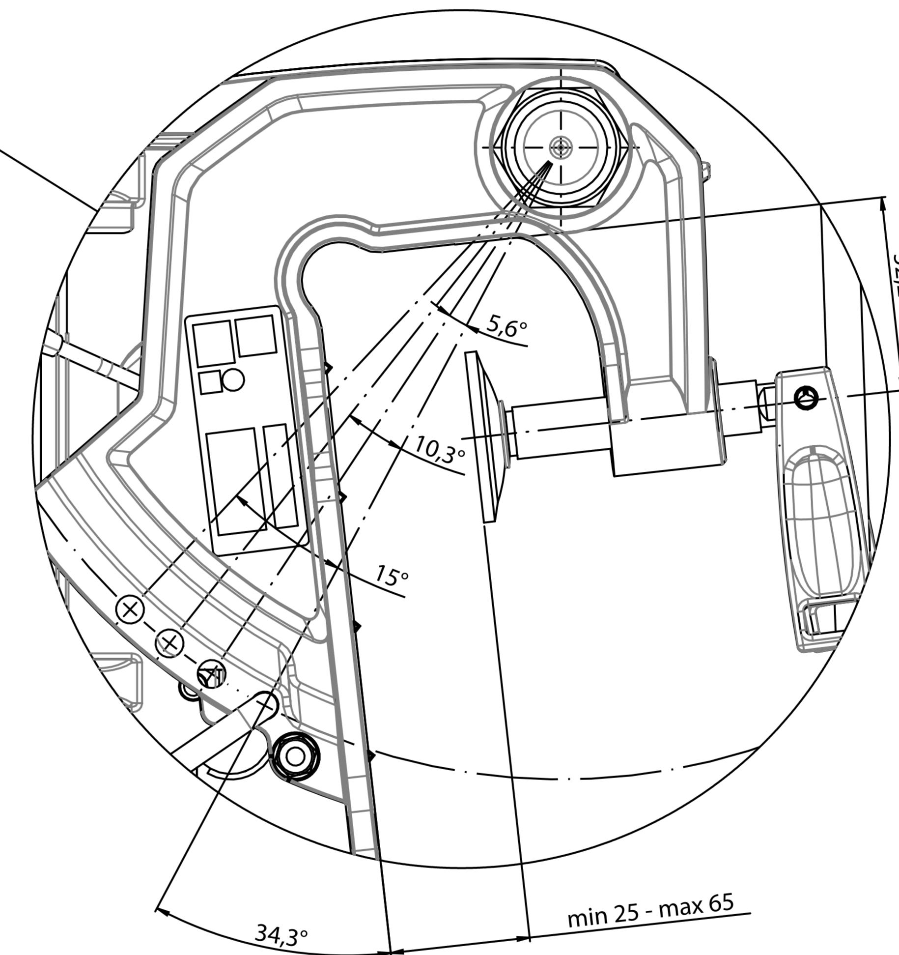
DETAIL Z MAßSTAB 1 : 1
